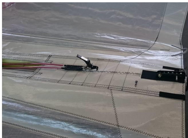
Figure 5-2 : Cheminement des câbles d'étarquage
